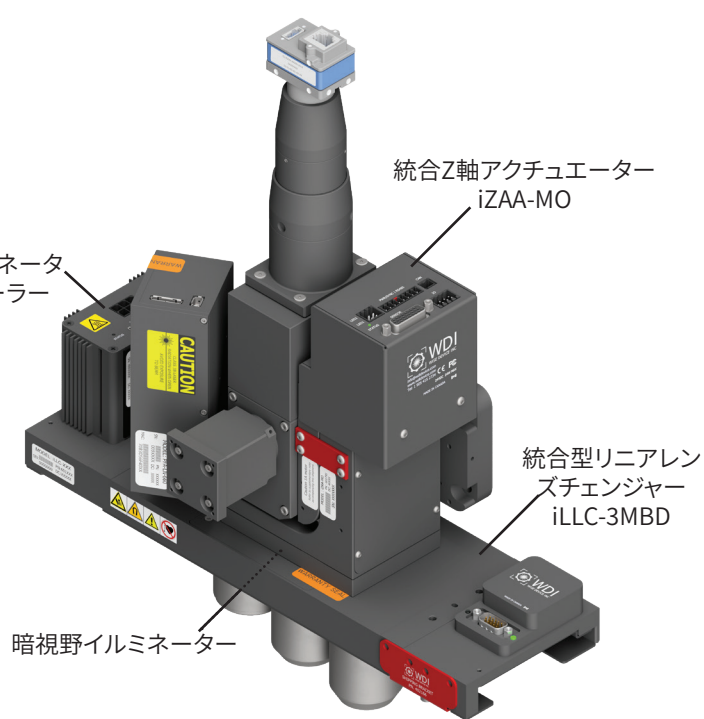
複数対物レンズシステム
