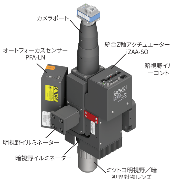
単一对物レンズシステム
