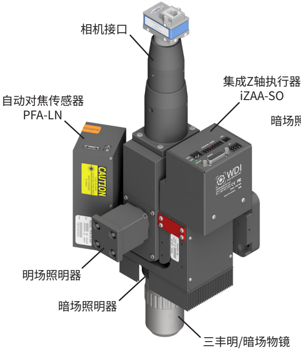
单物镜系统
